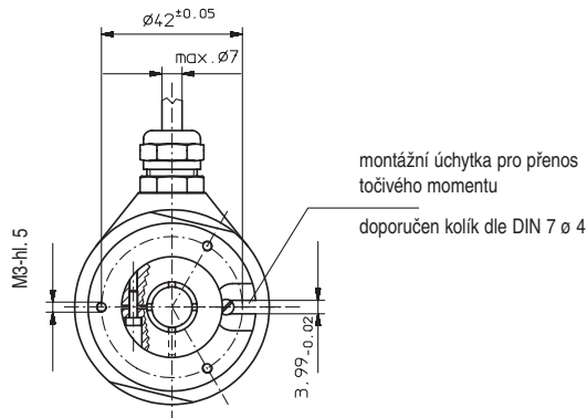
příruba typ 1
