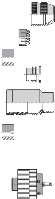
Obr. 2: Stínění umístěno, vodiče s krimpovacími trubičkami
