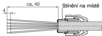
Obr. 2: Stínění umístěno, vodiče s krimpovacími trubičkami
