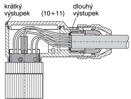
Obr. 6: Smontovaný konektor
