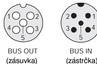
Obr. 4-1: Osazení pinů BKS na BTL...S 94
