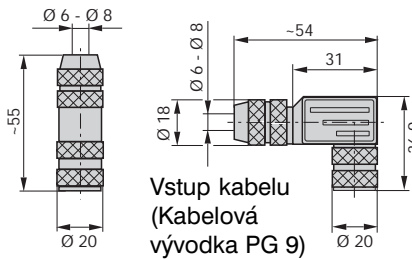
Obr. 4-3: Konektory (zástrčka) pro BUS IN
