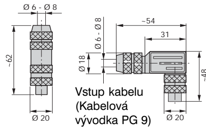
Obr. 4-4: Konektory (zásuvka) pro BUS OUT
