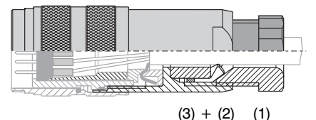
Obr. 6: PG šroubení zašroubováno, konektor kompletně smontován
