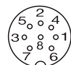
Obr. 3: Tělo zástrčky (8)
