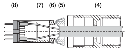
Obr. 4: Vodiče připájeny a distanční trubička namontována
