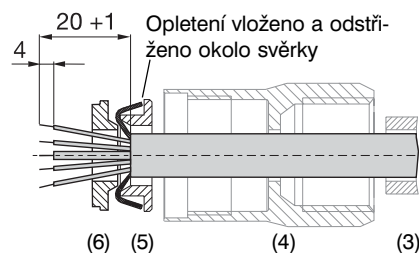
Obr. 2: Opletení sevřeno a vodiče odizolovány a pocínovány
